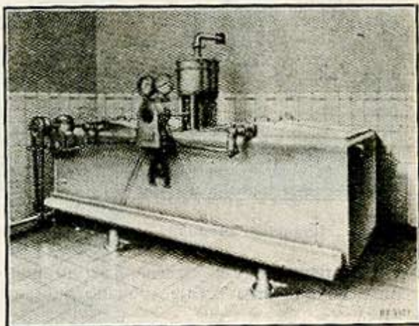
Пастеризатор за нижу температуру
