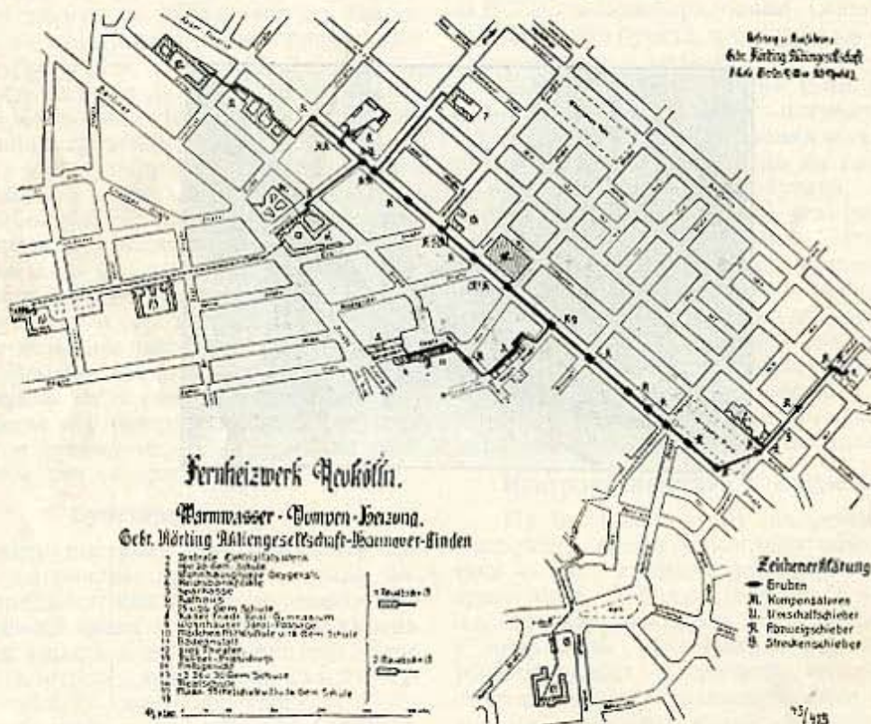
План мреже за грејање на даљину једног дела града (Берлин—Најкелн). Прикључници за поједине зграде означени су тачкама.
