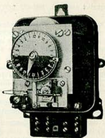
3. Аутоматски часовник за укључивање цифреника.
