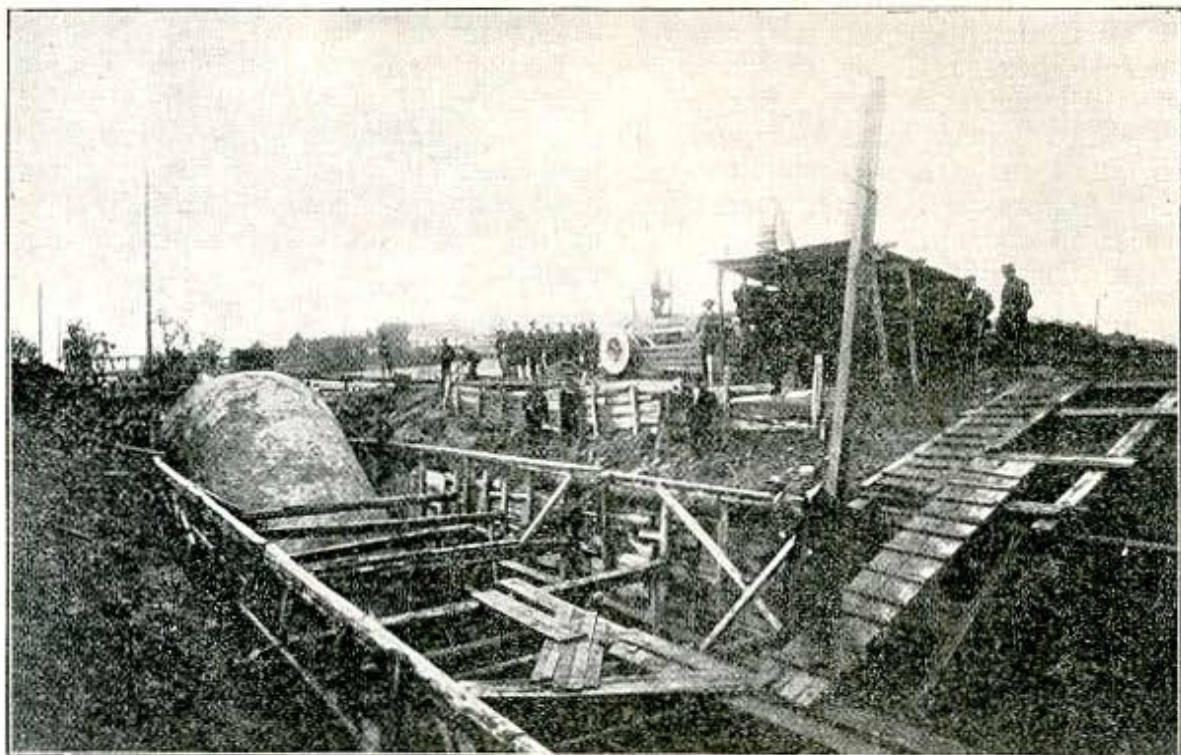
Сифон испод будућег корита Топчидерске Реке
